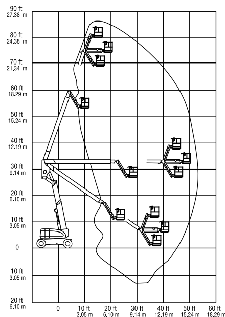
JLG 800 AJ
