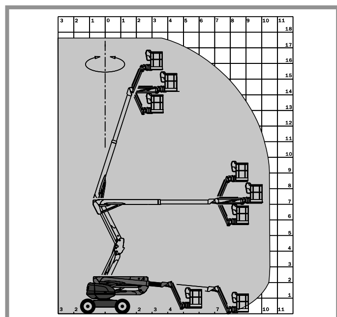
Manitou 180 ATJ
