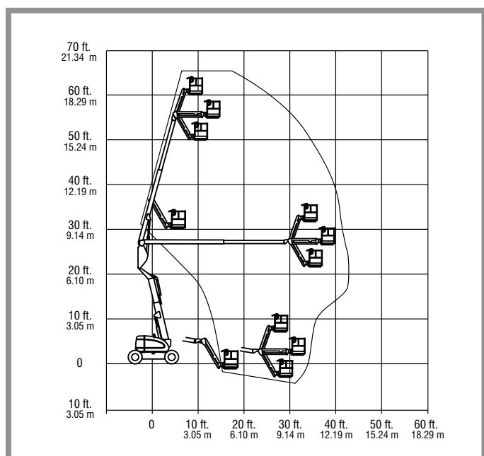
JLG 600 AJ
