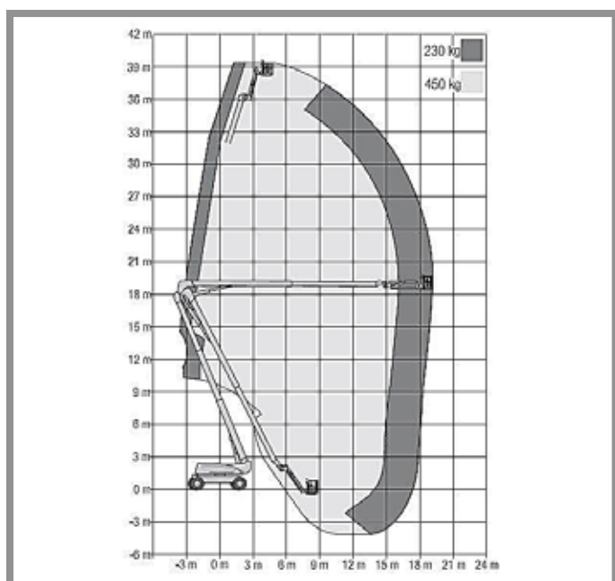
JLG 1250 AJP
