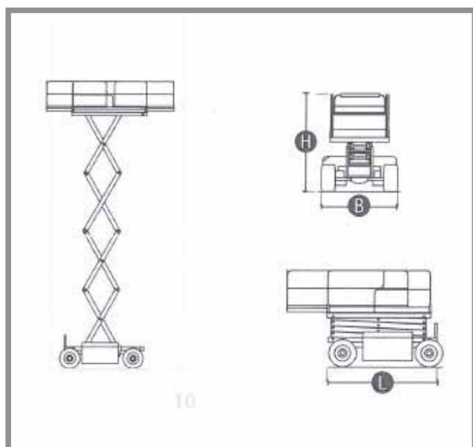
JLG 3394 RT
