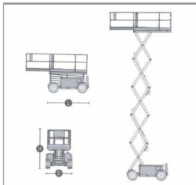
Genie 2668 RT
