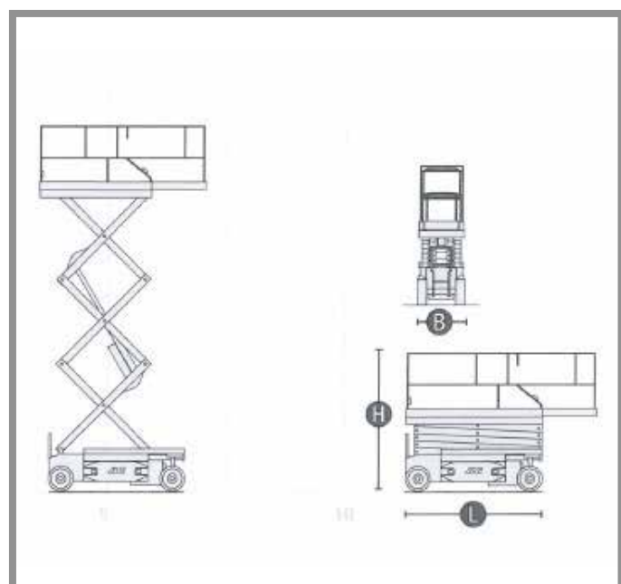
JLG 1930 ES
