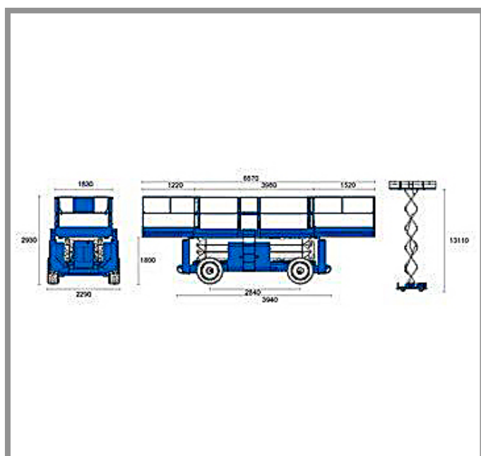
Genie 4390 GS
