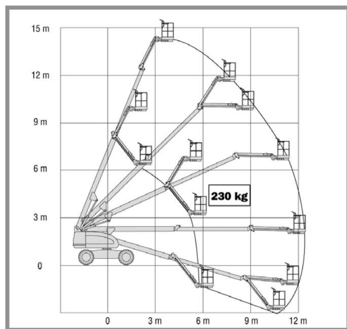
JLG 460 SJ
