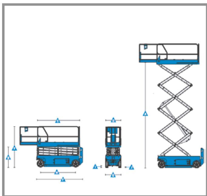
Genie GS 4047
