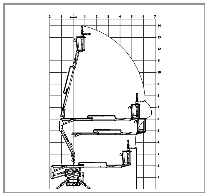
Hinowa 14,7 bælte
