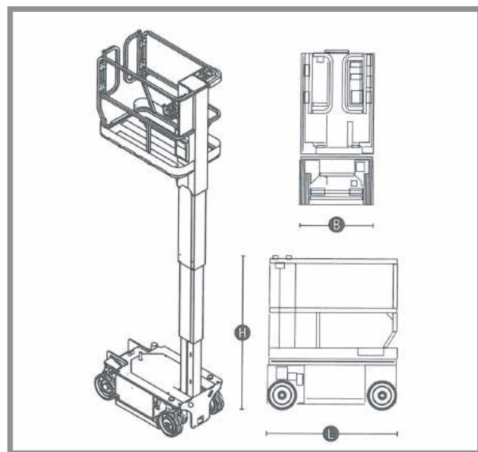
JLG 1230 ES
