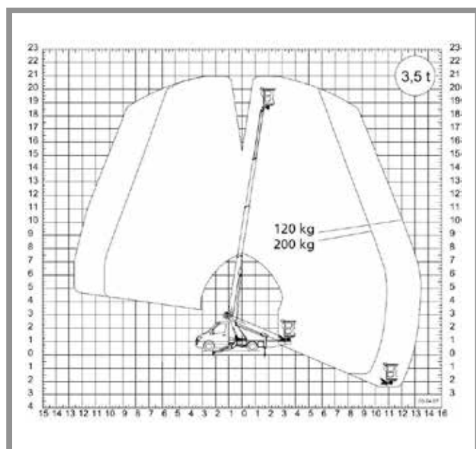
Palfinger TM21B
