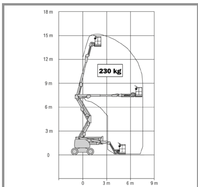
JLG 450 AJ
