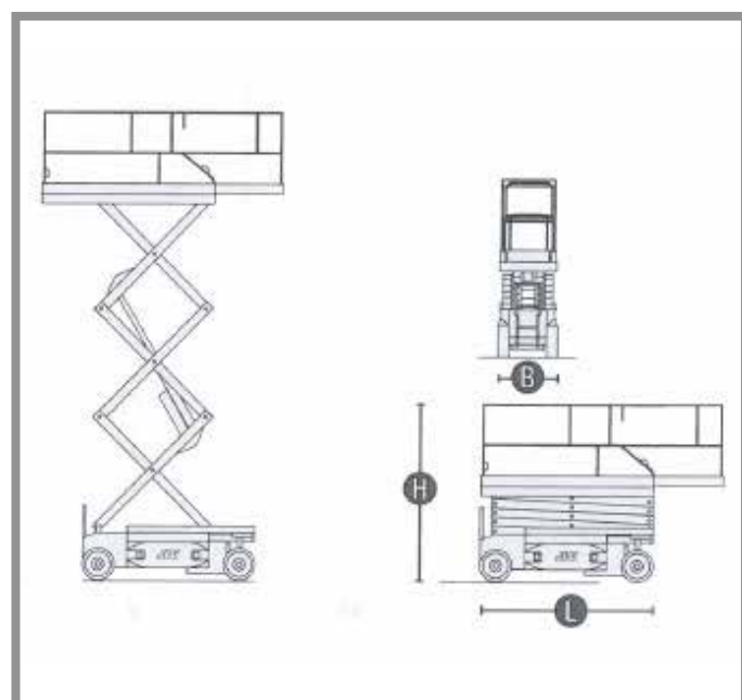
JLG 3246 ES
