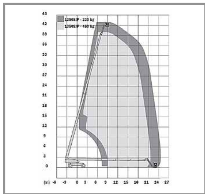
JLG 1350 SJP
