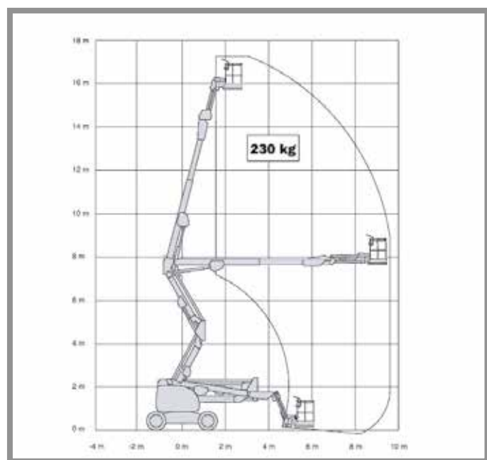
JLG 510 AJ
