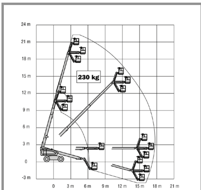
JLG 660 SJ
