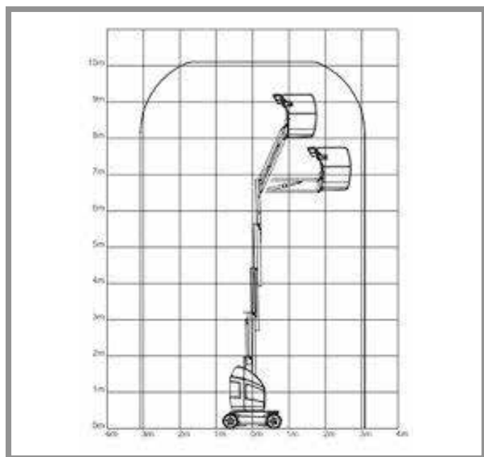
JLG Toucan 800
