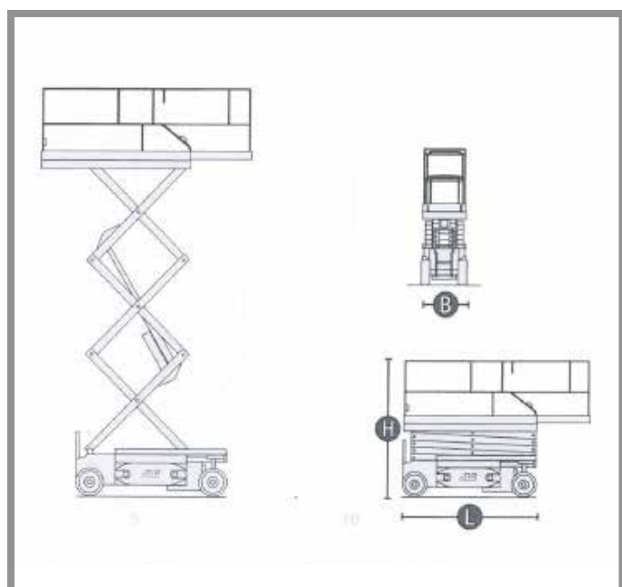
JLG 2630 ES
