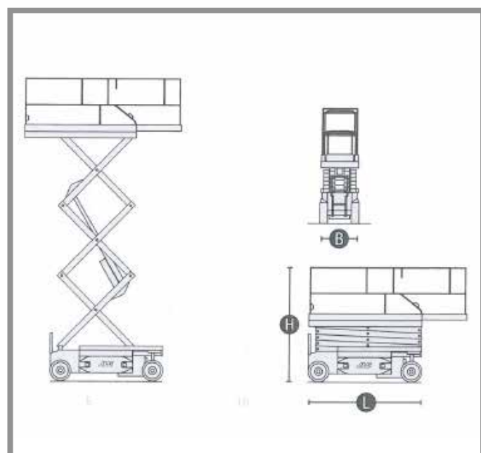
JLG 2646 E
