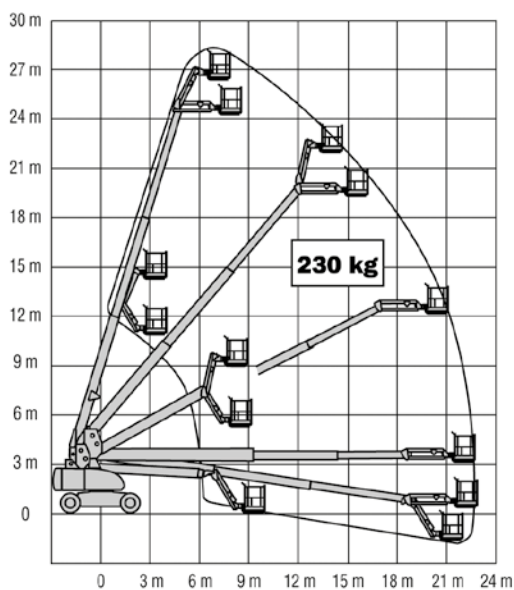
JLG 860 SJ
