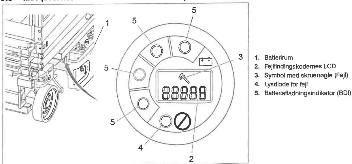
Figur 3-4. MDI (Digital multifunktionsindikator)
