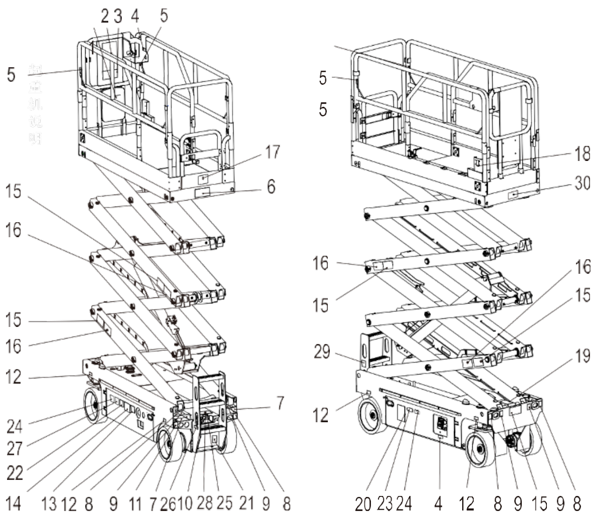
Figur 3-6 Mærkatplacering 6 ( ZS0607HD/ZS0607HD-Li/ZS0607DC/ZS0607DC- Li )
