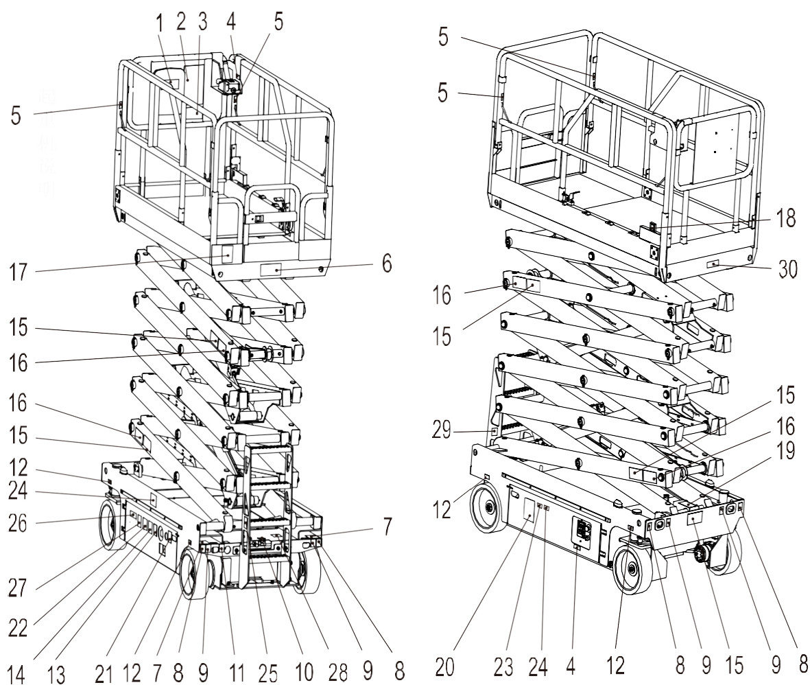
Figur 3-2 Mærkatplacering 2 ( ZS1212HD/ZS1212HD-Li/ZS1212DC/ZS1212DC- Li )
