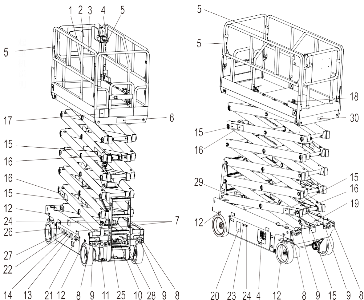
Figur 3-1 Mærkatplacering 1 ( ZS1414HD/ZS1414HD-Li/ZS1414DC/ZS1414DC- Li )
