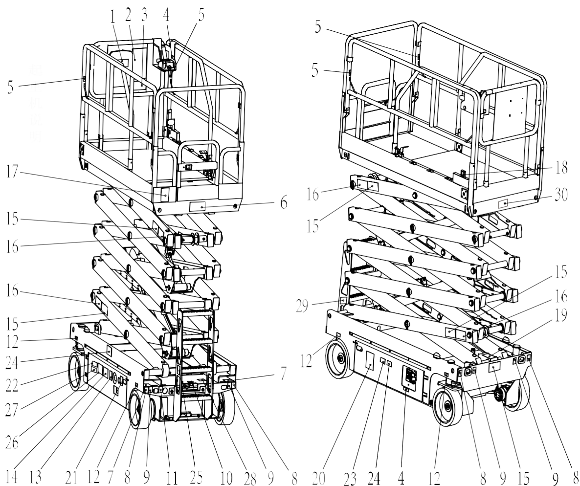
Figur 3-3 Mærkatplacering 3 ( ZS1012HD/ZS1012HD-Li/ZS1012DC/ZS1012DC- Li )
