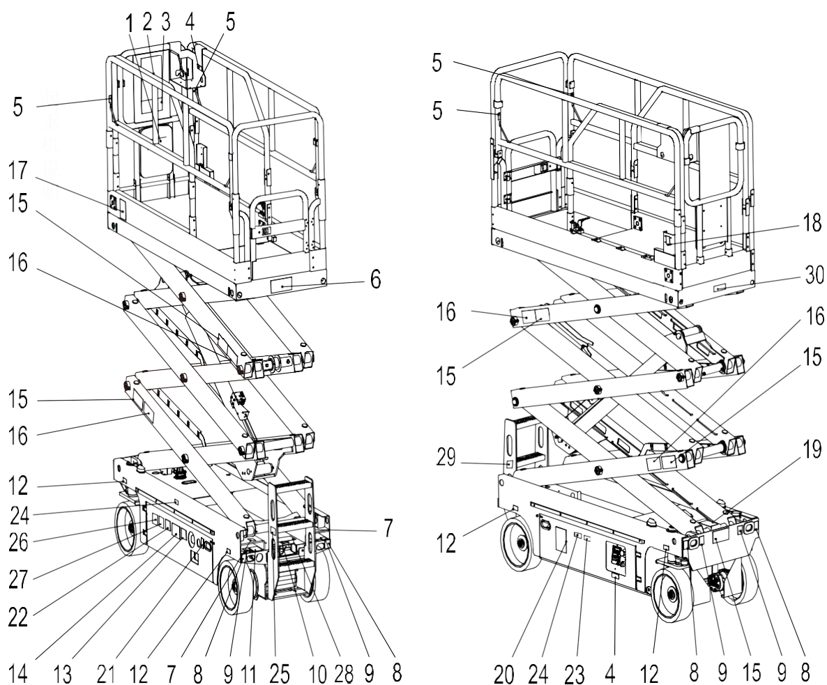
Figur 3-5 Mærkatplacering 5 ( ZS0608HD/ZS0608HD-Li/ZS0608DC/ZS0608DC- Li )
