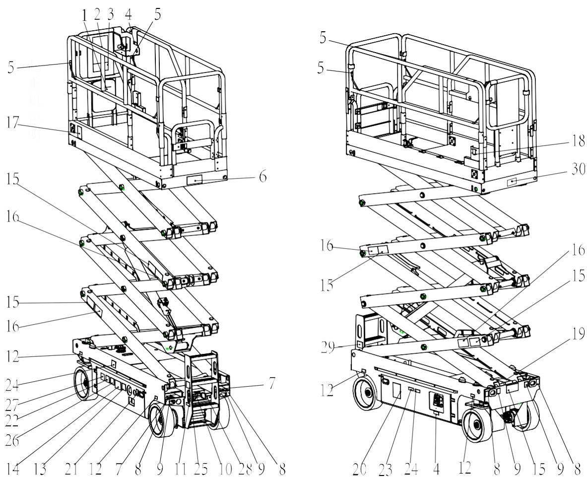
Figur 3-4 Mærkatplacering 4 ( ZS0808HD/ZS0808HD-Li/ZS0808DC/ZS0808DC- Li )
