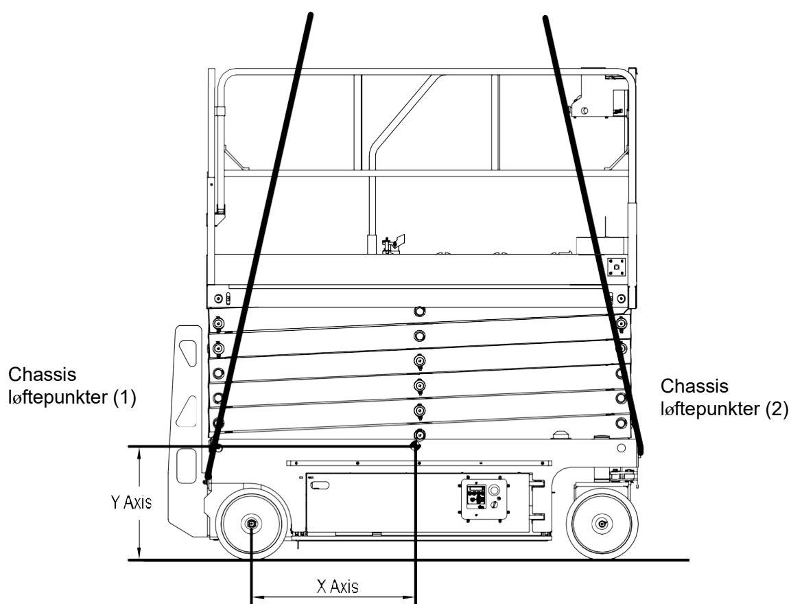
Figur 4-4 Tyngdepunkt
