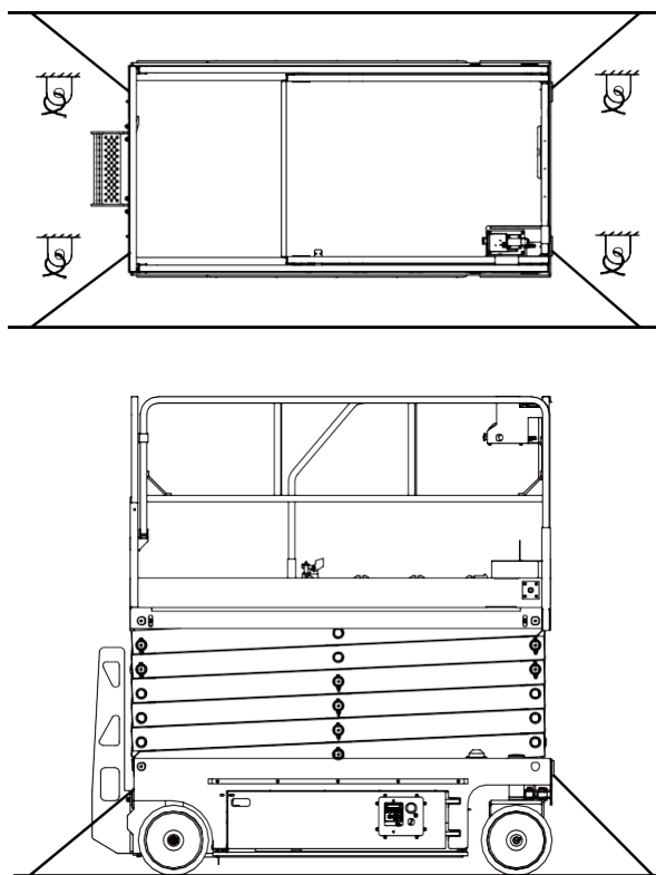
Figur 4-2 Fastspændingspunkter
