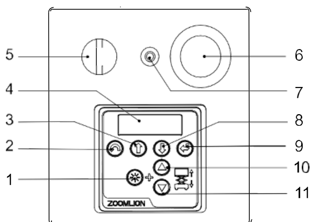
Figur 2-4 Elektronisk betjeningspanel
