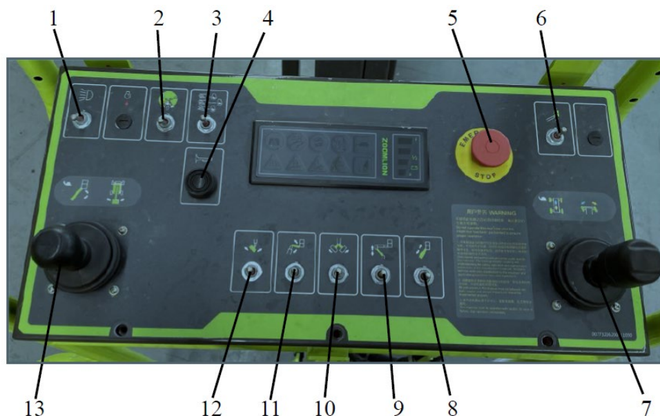
Figur 2-9 Platforms kontrolpanel (Kun det kontaktnummer, der svarer til det eksisterende funktion er identificeret.)
