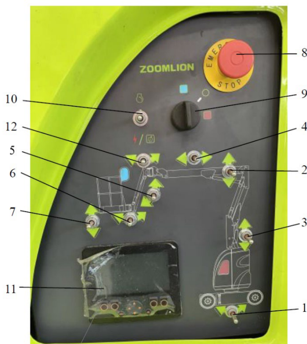
Figur 2-2 Kontrolpanel på jorden
