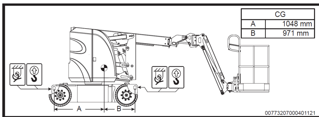
Figur 4-5 Løfte og sikrings instruktioner
