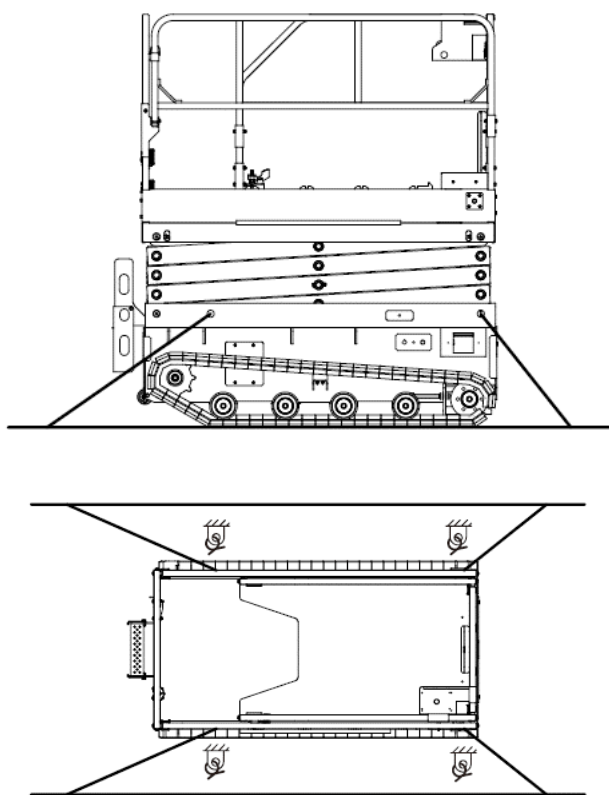
Figur 4-3 Fastspændingspunkter
