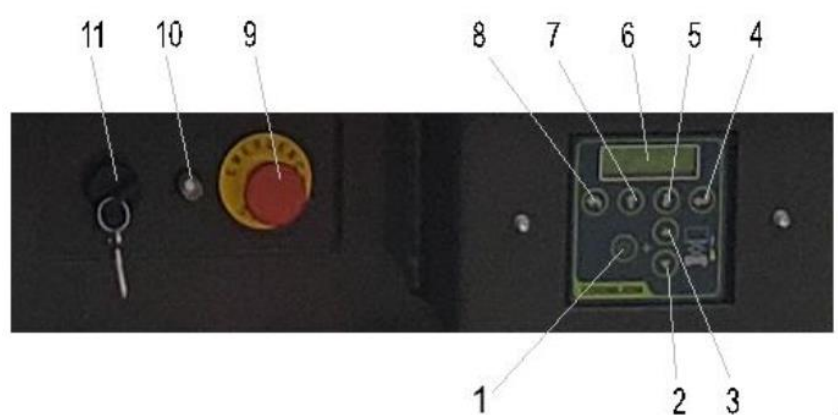
Figur 2-2 Elektronisk jordbetjeningspanel
