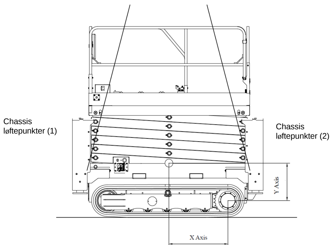
Figur 4-4 Tyngdepunkt
