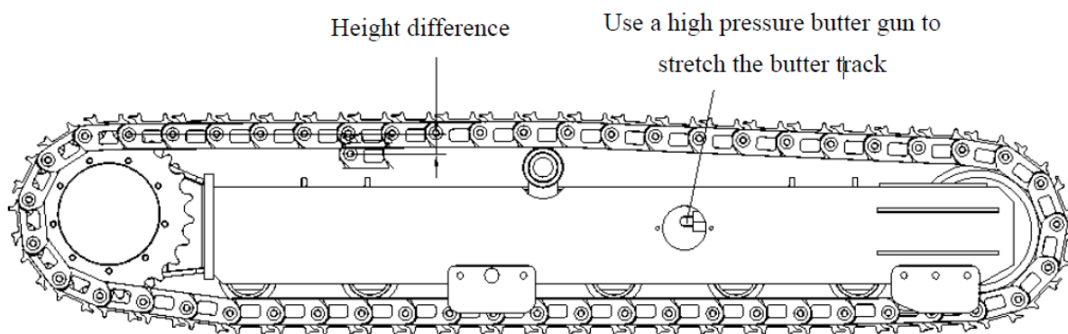
Figur 5-5 ZS1216C bæltespændingsdiagram
