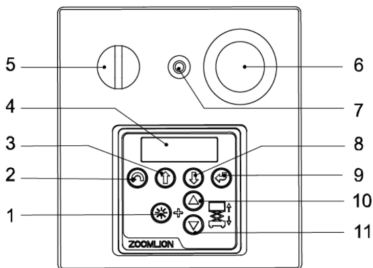
Figur 4-1 Elektronisk kontrolpanel
